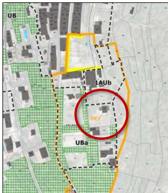
// Modification n°1
